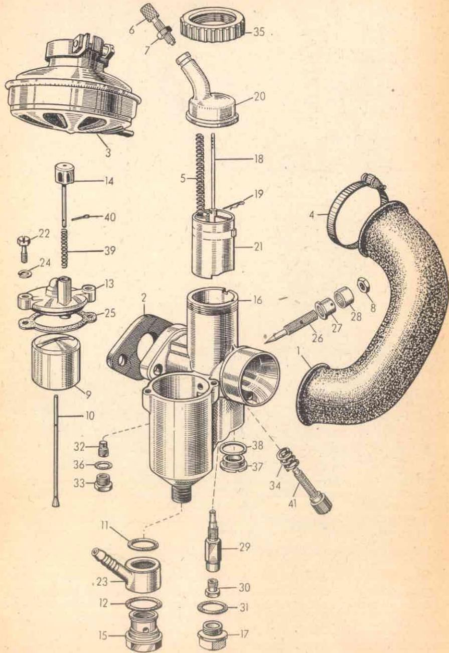
Bing-Vergaser
