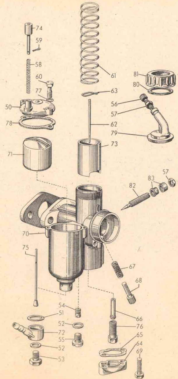
SAWE-Vergaser
